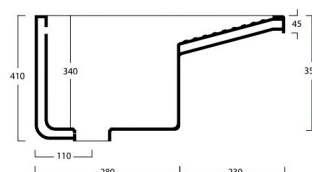
Sezione / Section
