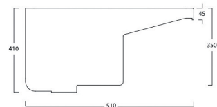
Sezione / Section
