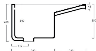
Sezione / Section
